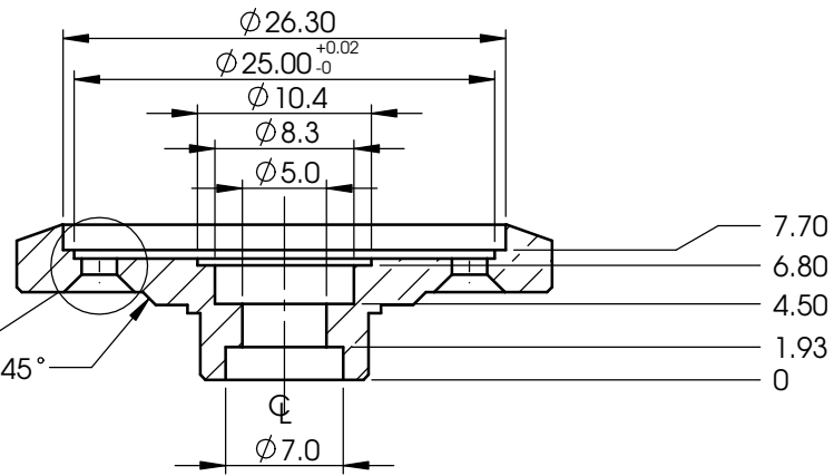
剖面圖 A-A
