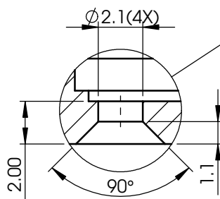
細部放大圖 C 比例 4 : 1
